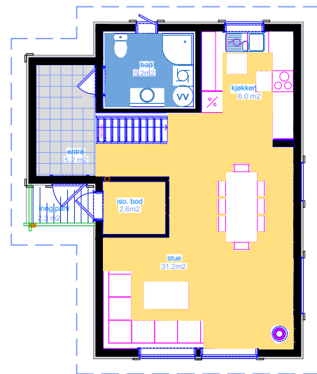
Plan 1.etg
